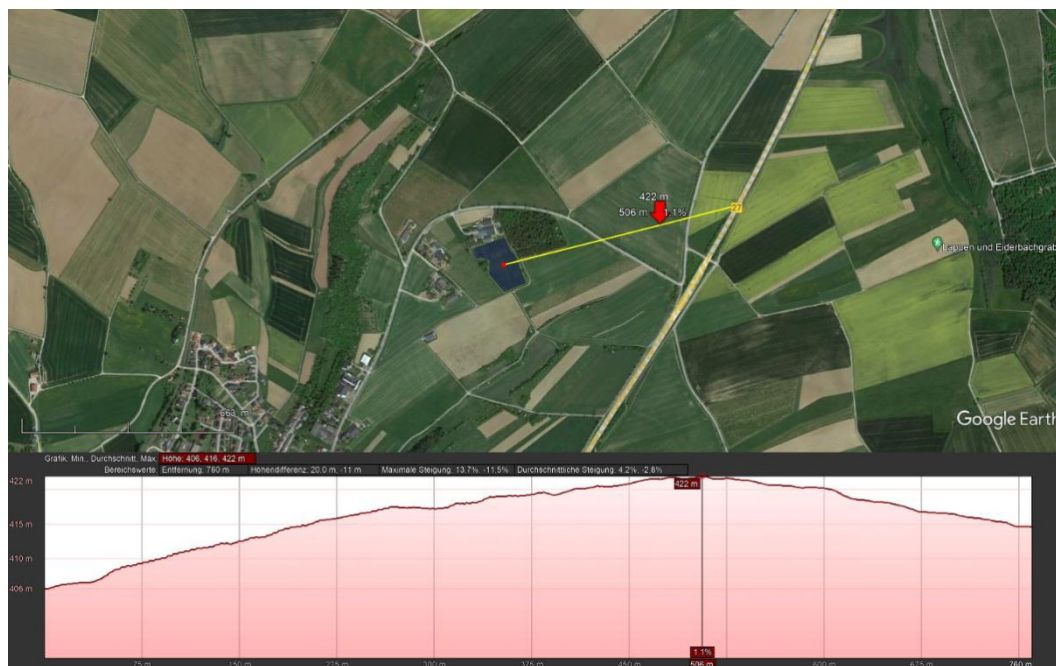
Abbildung 6: Höhenprofil zwischen Photovoltaikanlage und Punkt B5
